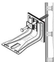
Ventilirana fasada (HPL, ACP, kamen, staklo...)
